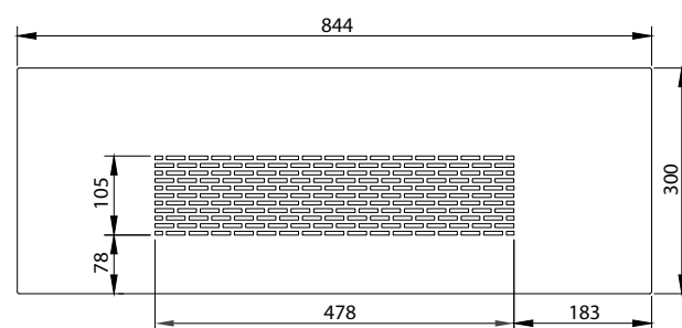
Panel ochronny środkowy z otworami pod zamek z blokadą/klucz/wkładkę
