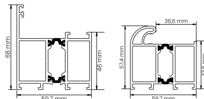
PROFIL NAŚWIETLA PROFIL OŚCIEŻNICY ALU/54
