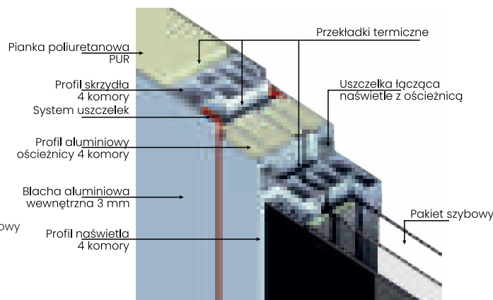
PROFIL OŚCIEŻNICY
