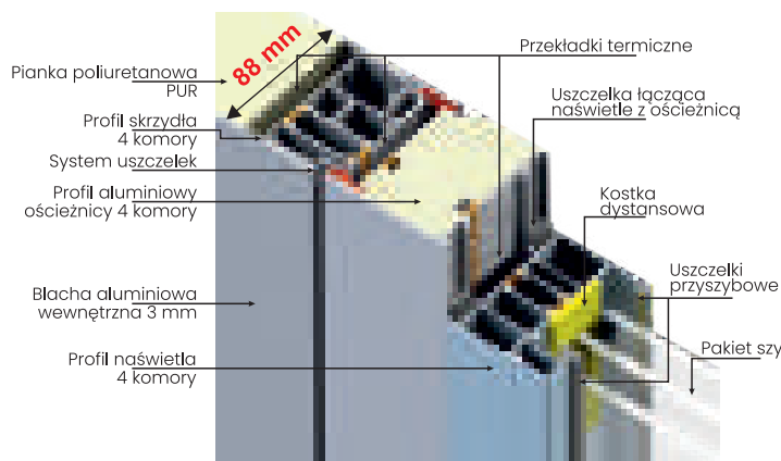
PROFIL OŚCIEŻNICY
