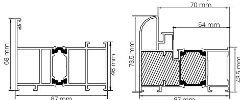
PROFIL NAŚWIETLA PROFIL OŚCIEŻNICY ALU/90
