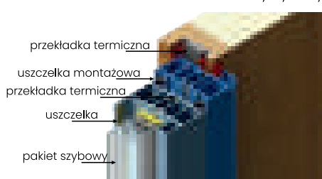
PROFIL NAŚWIETLA PROFIL OŚCIEŻNICY ALU/75
