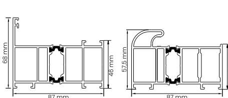
PROFIL NAŚWIETLA PROFIL OŚCIEŻNICY ALU/75
