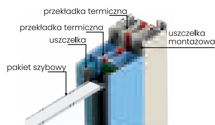
PROFIL NAŚWIETLA PROFIL OŚCIEŻNICY ALU/54
