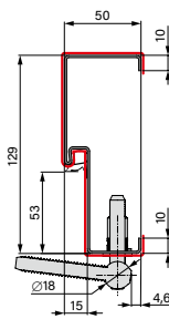
OŚCIEŻNICA STALOWA
