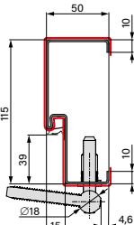
OŚCIEŻNICA STALOWA
