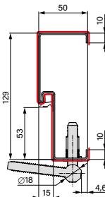
OŚCIEŻNICA STALOWA
