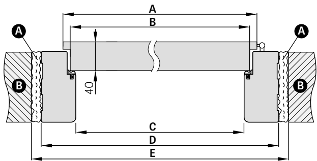
SCHEMAT OŚCIEŻNICY STAŁEJ BASIC
