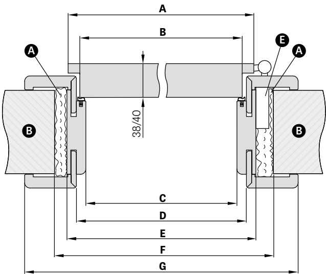
SCHEMAT OŚCIEŻNICY REGULOWANEJ
