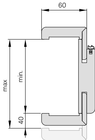
ZAKRES REGULACJI OŚCIEŻNICY REGULOWANEJ
