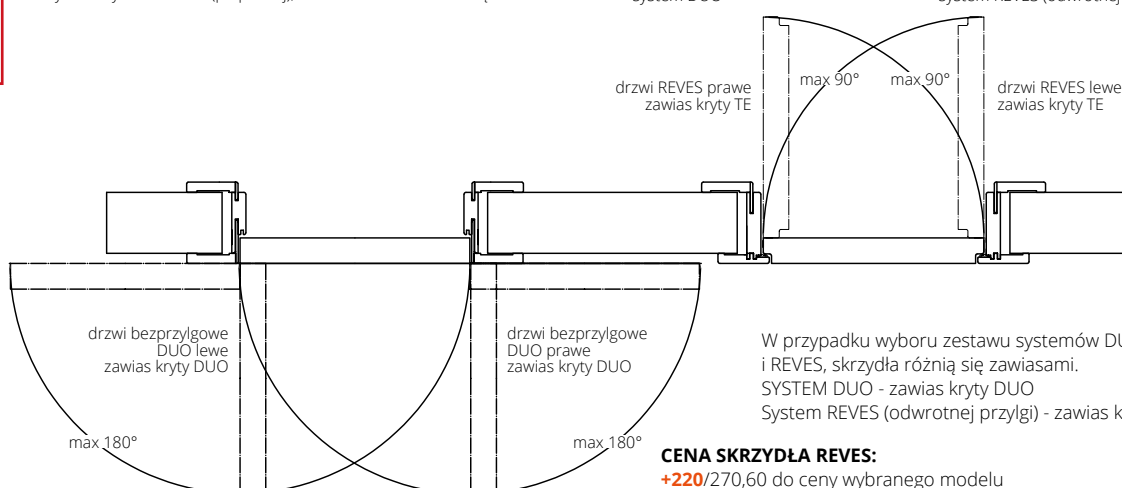
zawias kryty TE, kolor srebrny - system REVES (odwrotnej przyłgi)
