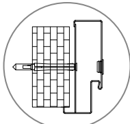
otwór montażowy kotwy w centrum profilu na persi ościeżnicy
