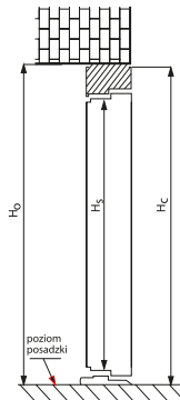
Wymiarowanie drzwi z ościeżnicą ALU HYBRID
