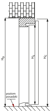
Wymiarowanie drzwi z ościeżnicą „11”, „12”, alumińowo-kompozytową oraz TERMO i TERMO PRESTIGE LUX
