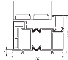
PROFIL NAŚWIEITŁA
