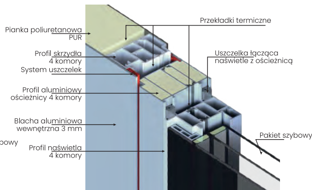
PROFIL OŚCIEŻNICY
