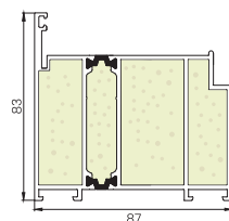
PROFIL OŚCIEŻNICY
