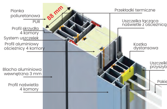
PROFIL OŚCIEŻNICY
