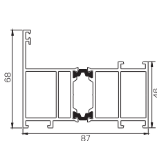
PROFIL NAŚWIEITŁA
