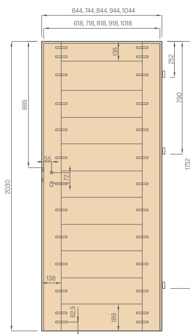
skrzydło przylgowe
