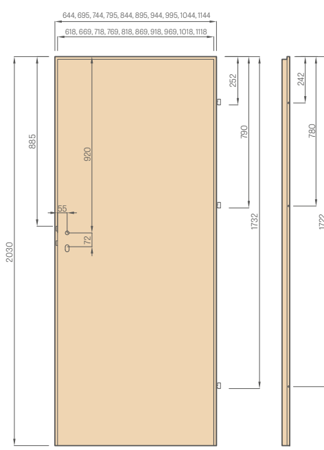
skrzydło przylgowe
