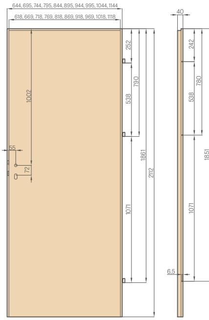
skrzydło przylgowe PL2112
